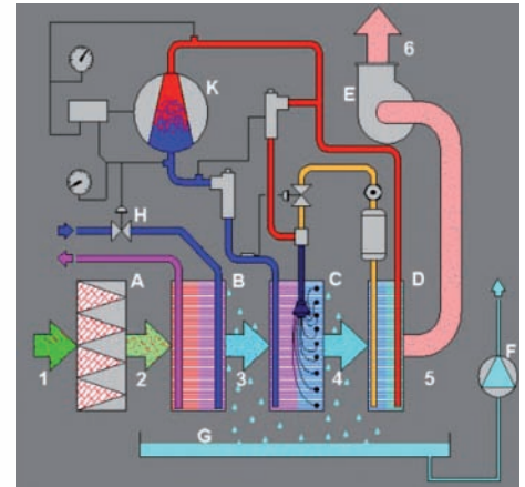
Über einen Filter wird Umgebungsluft angesaugt und in zwei Schritten gekühlt. Die Feuchtigkeit, die in Folge der Kondensation ausgeschieden wird, wird in einer Wanne gesammelt und über eine Pumpe aus dem Gerät gefördert. Die Wärme aus dem Verdampfer wird in den Kondensator geleitet, wo sie die vorgekühlte Umgebungsluft wieder auf 25 °C erwärmt. Diese wird anschließend über ein Rohrleitungssystem in eine abgeschottete Kabine eingeblasen, die die Form der Produktionsmaschine umgibt
